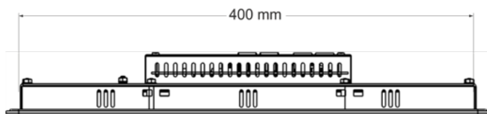
Maßblatt B-Primis ET-Pro 15
